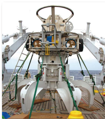
ファインダー付きパワーグラブ(FPG)
